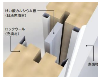
パネル構造
