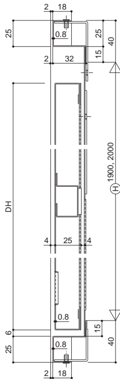
縦断面
