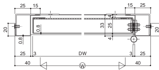
横断面
