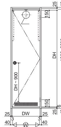
啓図
