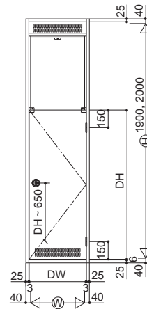
啓図
