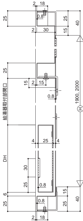
縦断面
