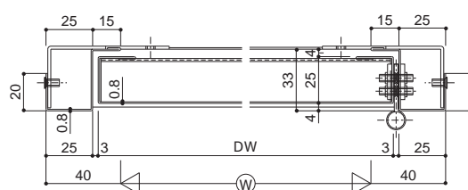
横断面
