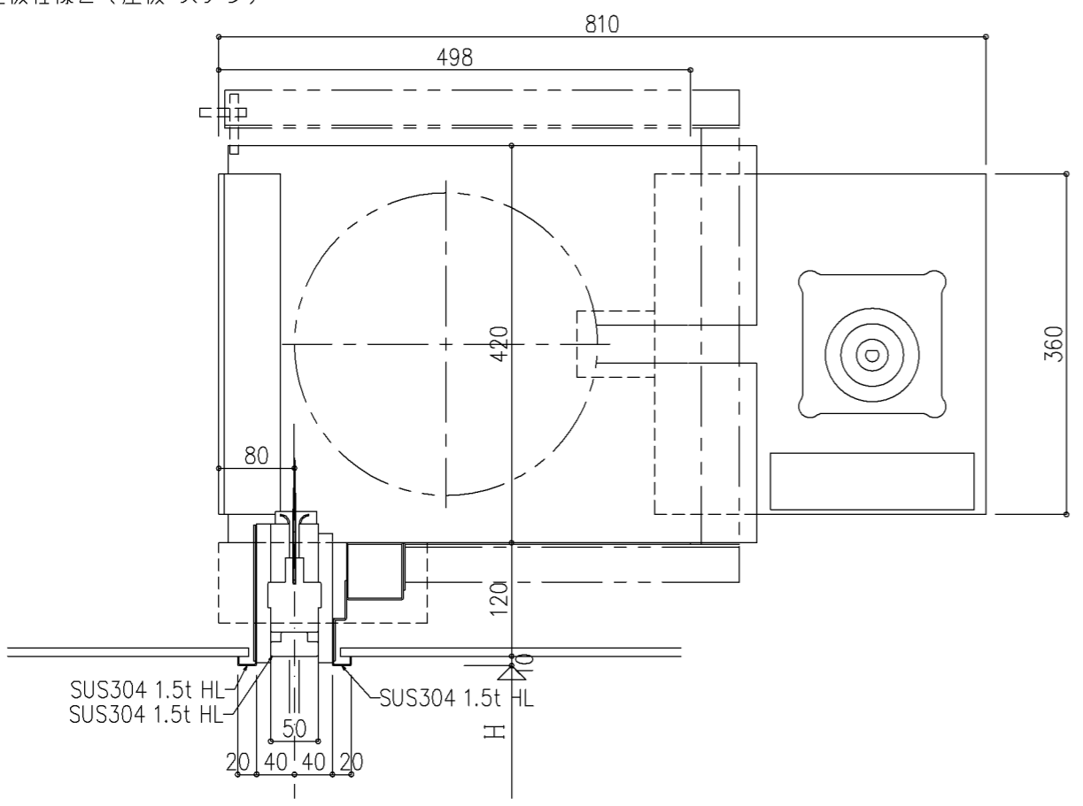
SD (一体形) 座板仕様2 (座板 ステン)
