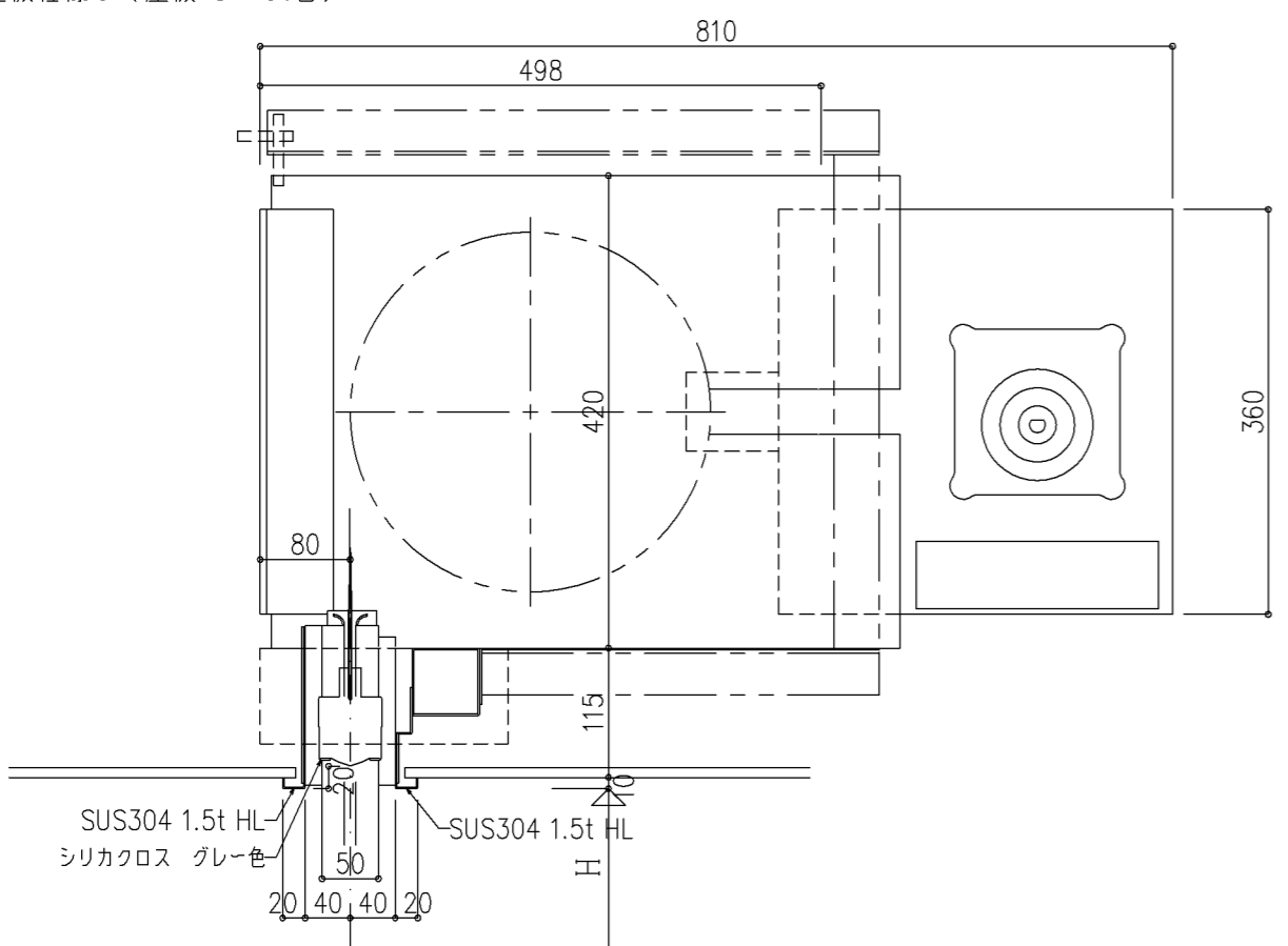
SD (一体形) 座板仕様1 (座板 クロス巻)
