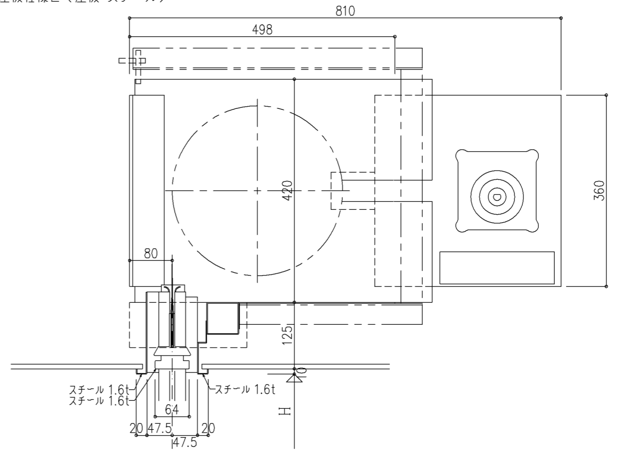
SD (一体形) 座板仕様2 (座板 スチール)
