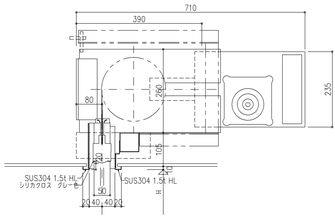
SD (一体形) 座板仕様1 (座板 クロス巻)
