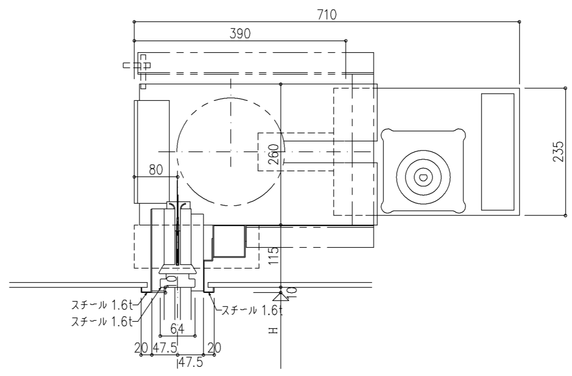
SD (一体形) 座板仕様2 (座板 スチール)
