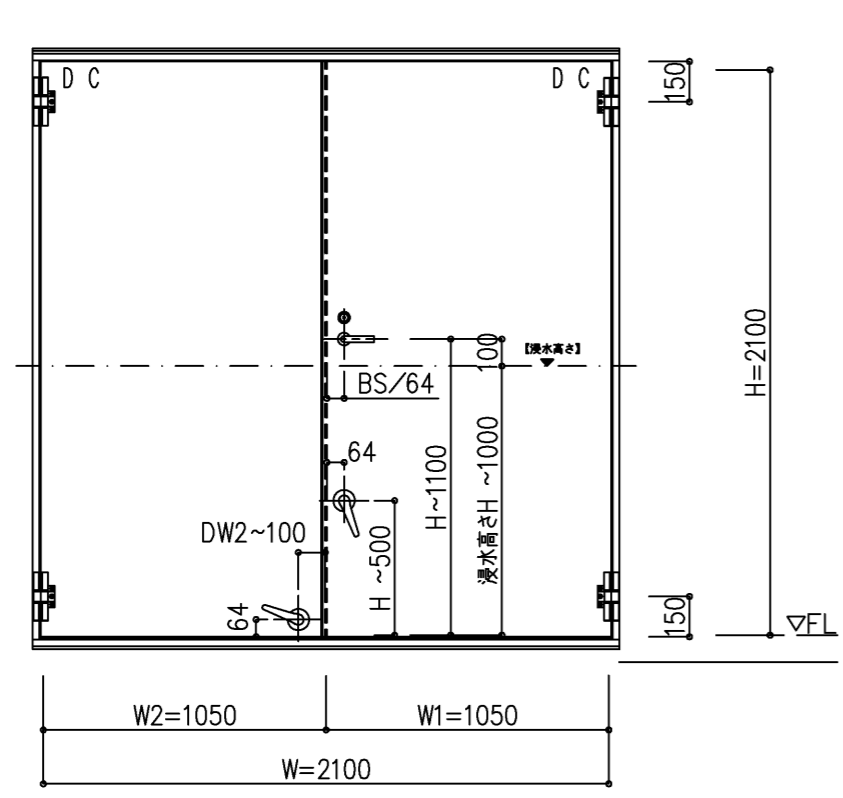
外観図
