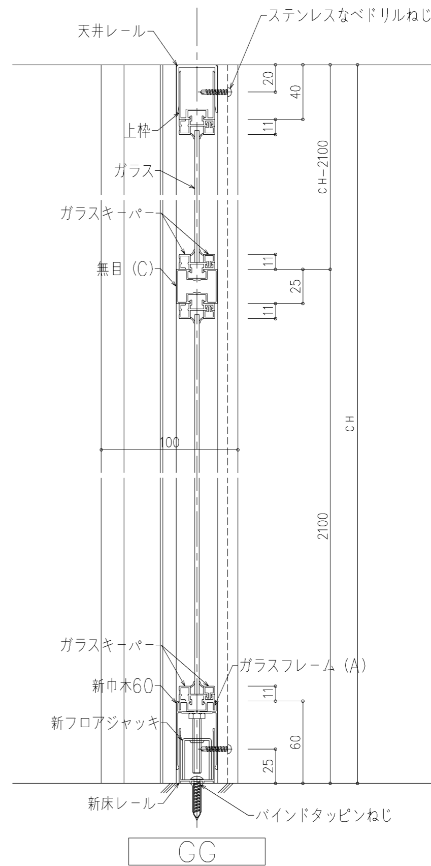
縦断面図
