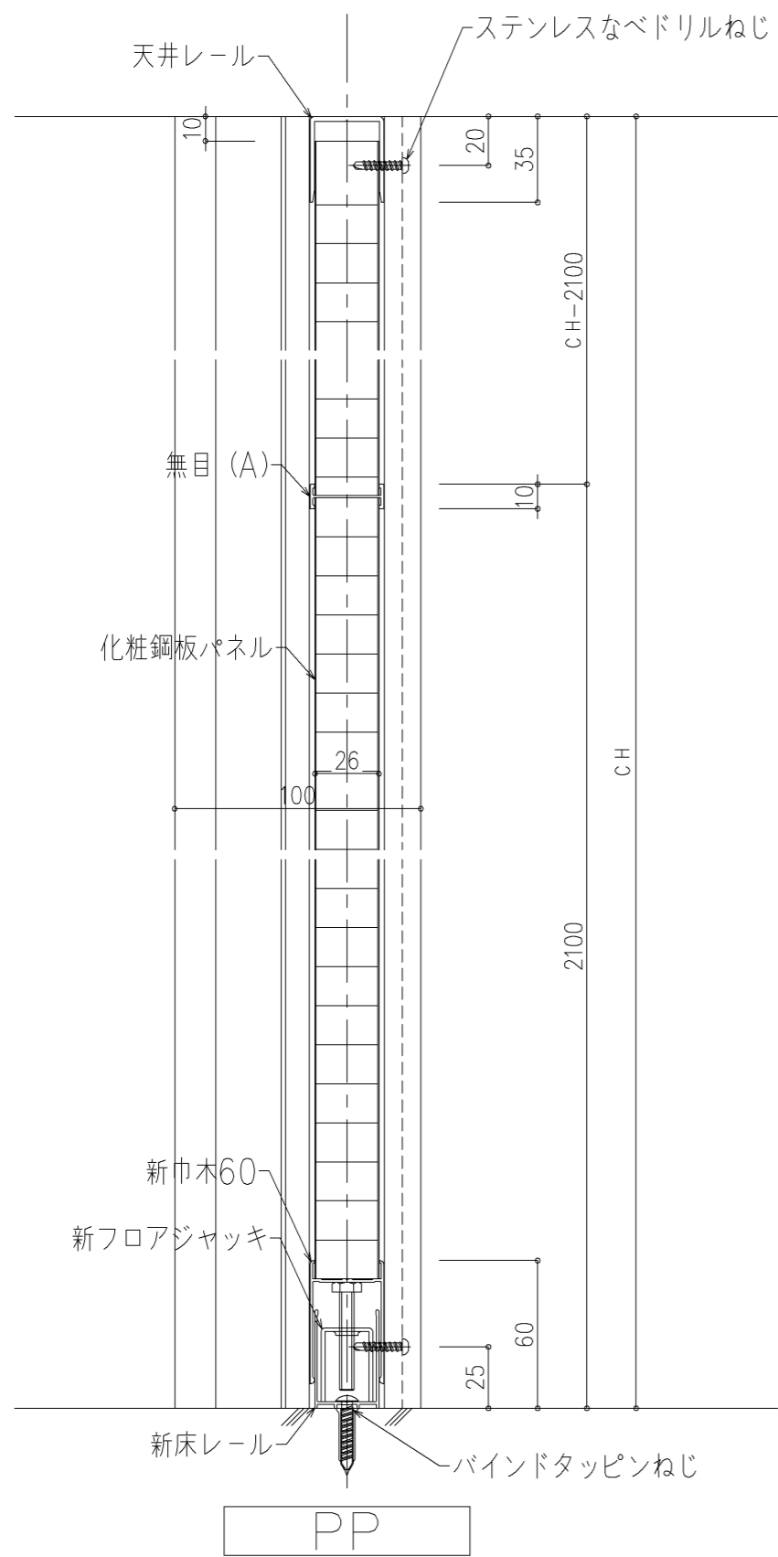
縦断面図
