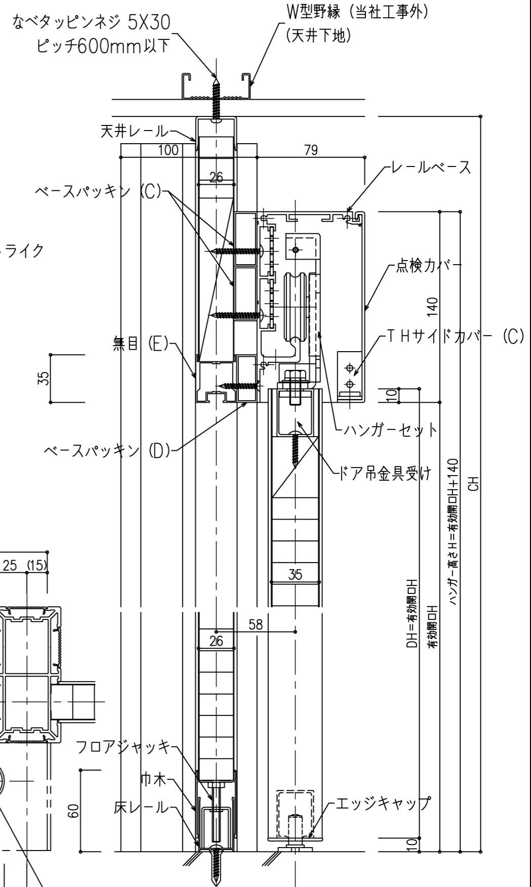
縦断面詳細図
