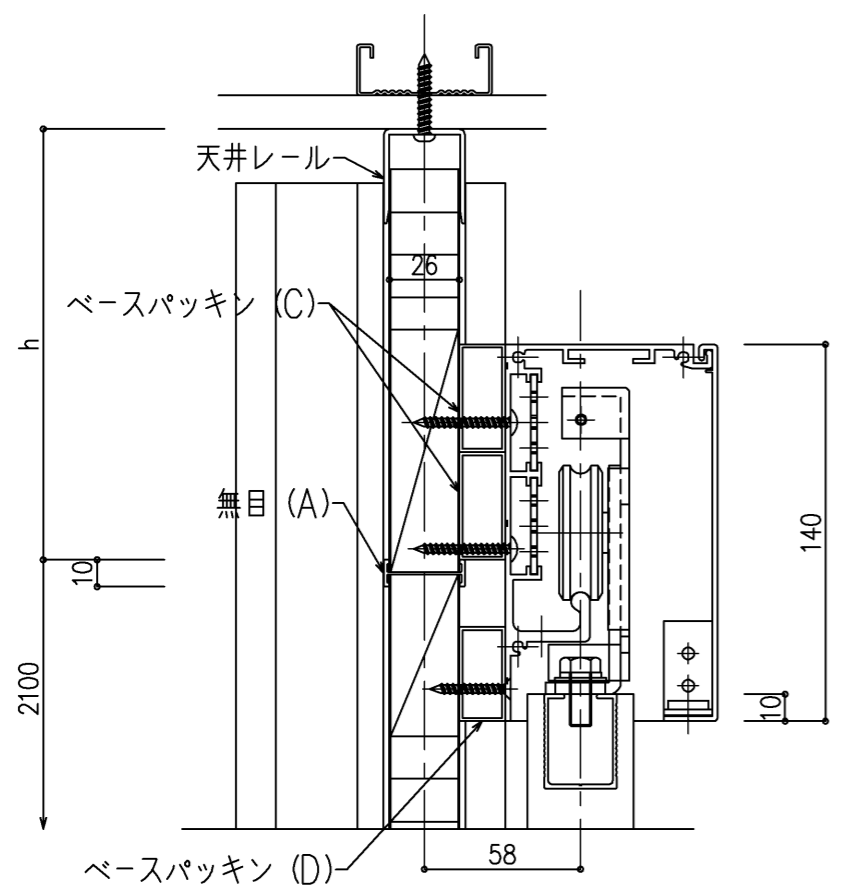
戸袋断面詳細図
