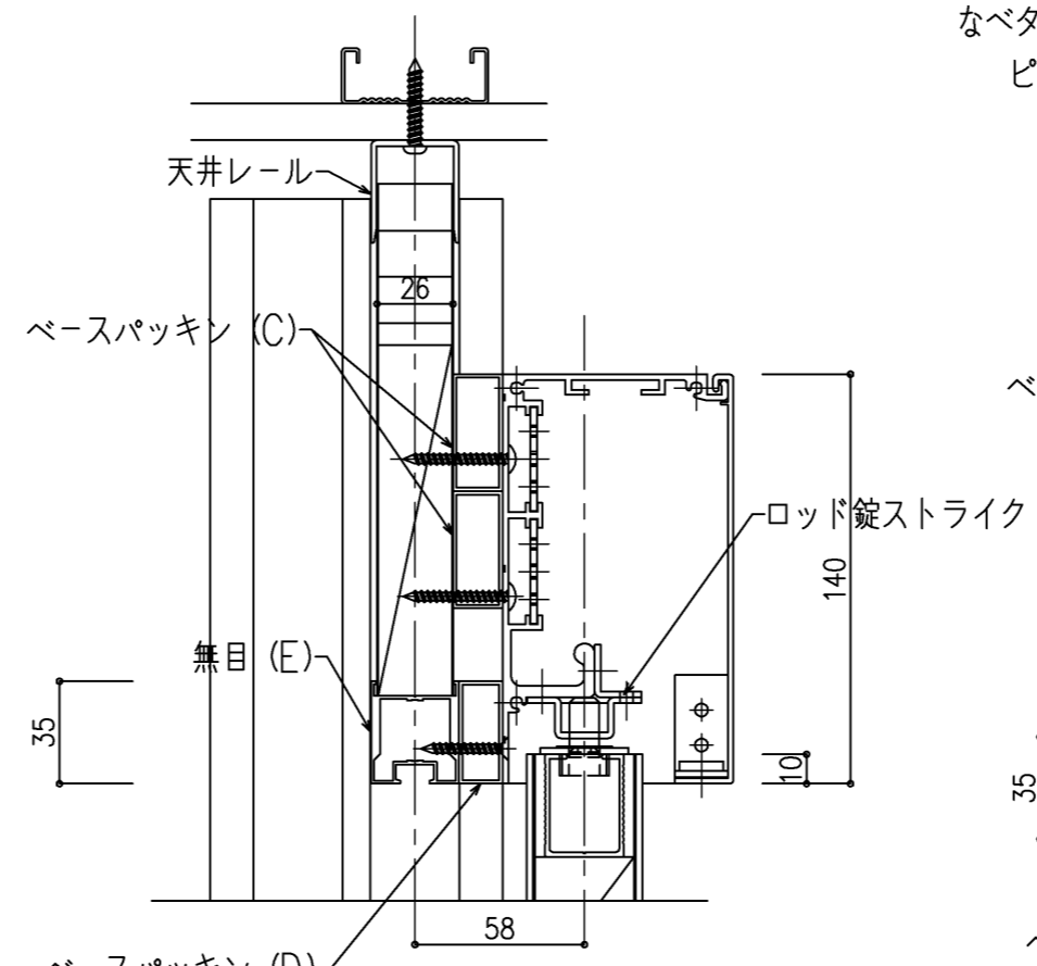
扉断面詳細図 (錠前)
