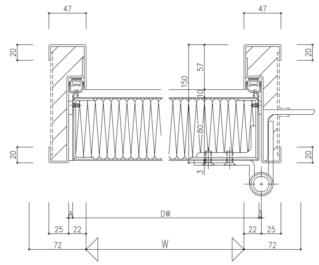
戸先チリ寸法
