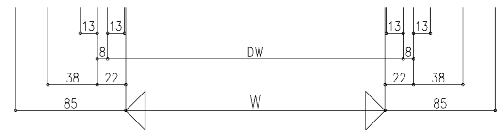
戸先チリ寸法
