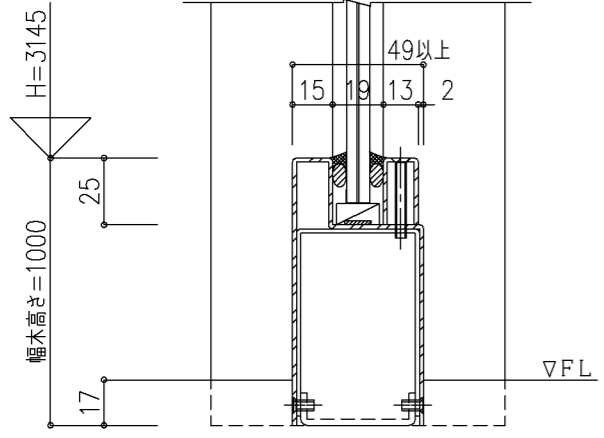
<幅木納まり>
