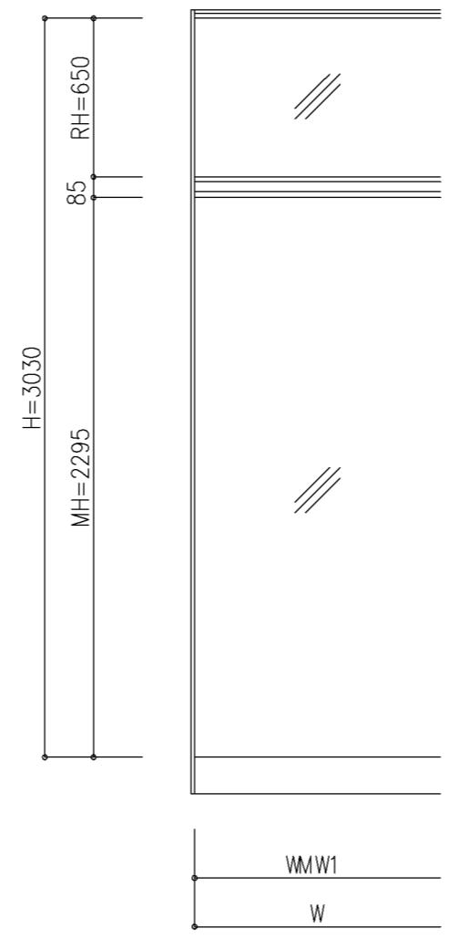
幅木納まり
