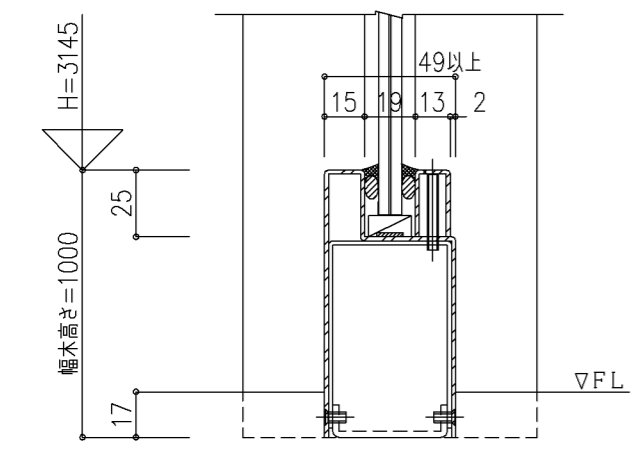
<幅木納まり>
