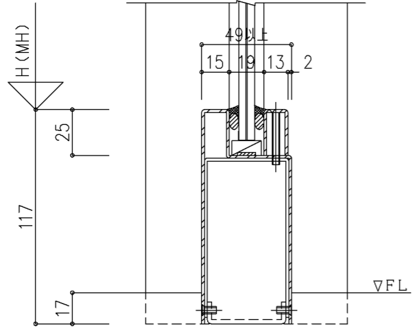
<幅木納まり>
