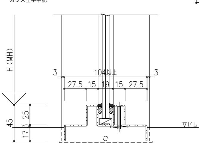
<床埋め込み納まり>
