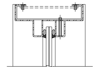
モルタル充填の場合の上枠
