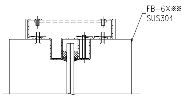
<FIX上枠>
