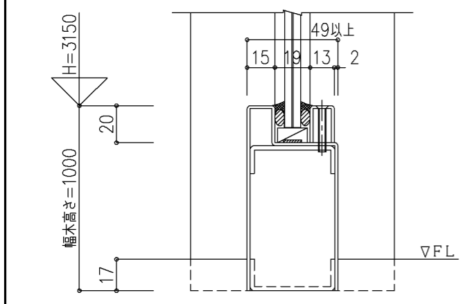
<幅木納まり>
