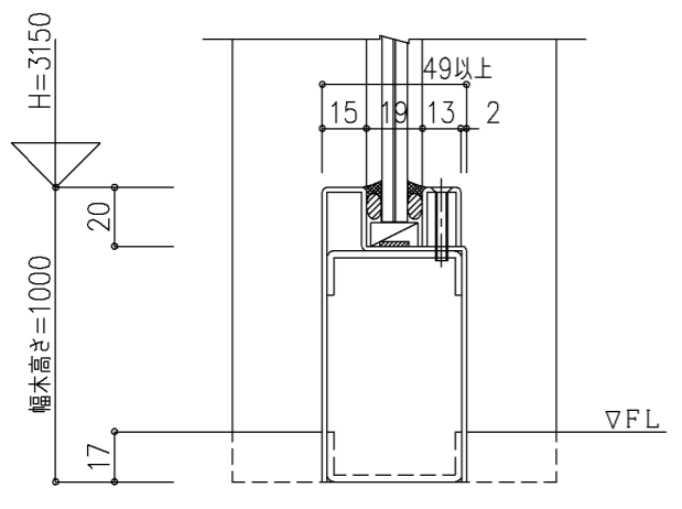
<幅木納まり>
