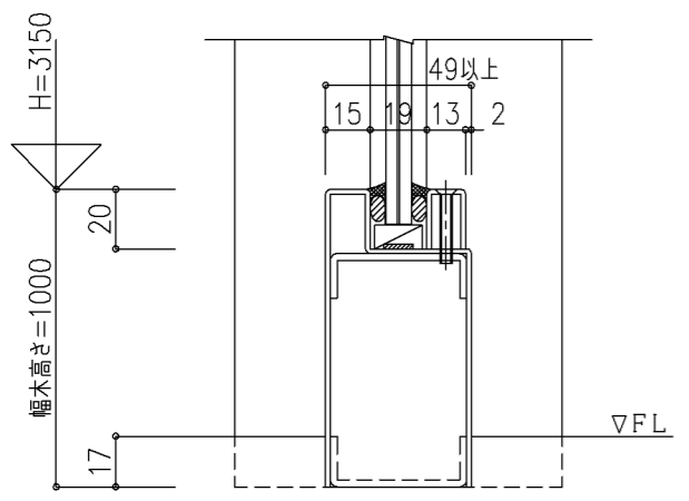
<幅木納まり>
