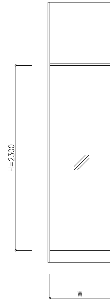
欄間幕板(上枠伸ばし)納まり
