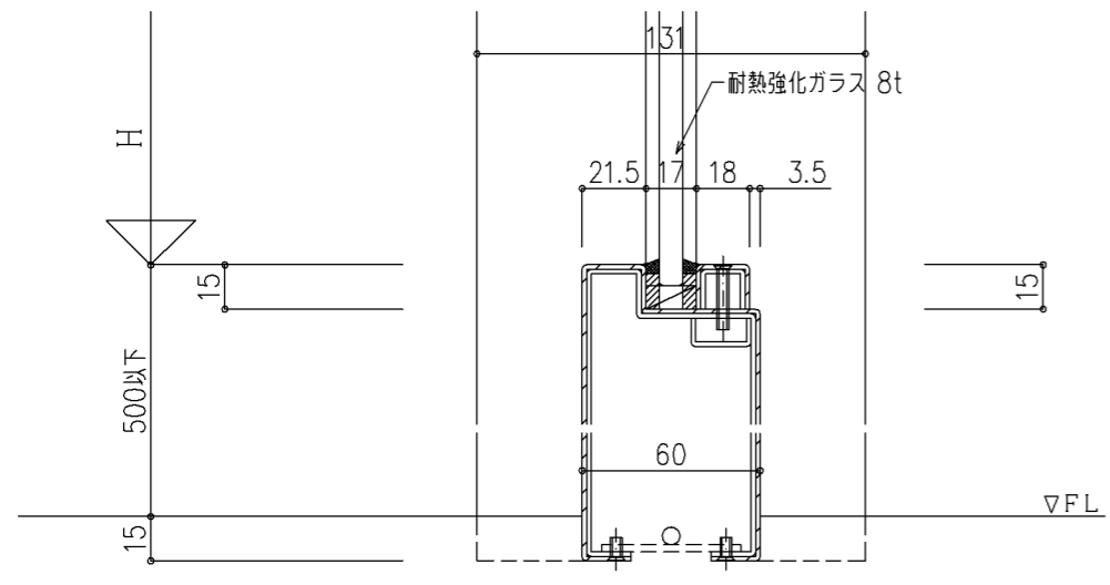
幅木納まり
