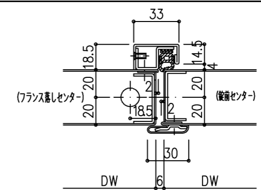
SAT枠 目板付外(R)
