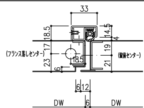
SAT枠 目板一体外(R)
