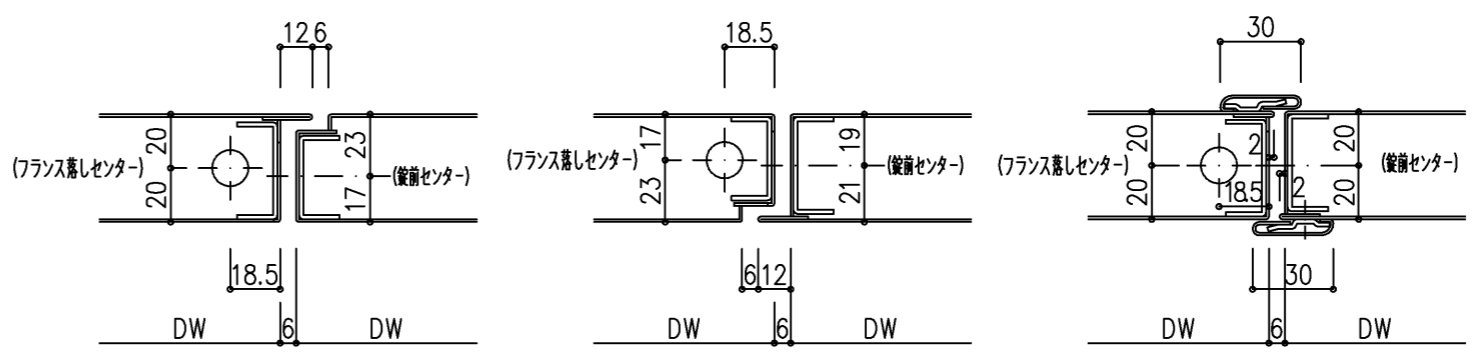
ST枠 目板一体 内開き外(R) ST枠 目板一体 外開き外(R) ST枠 目板付B外(R)
