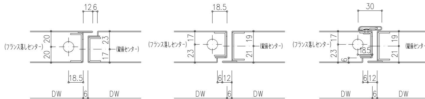
ST樑 目板一体 内開き(R)
