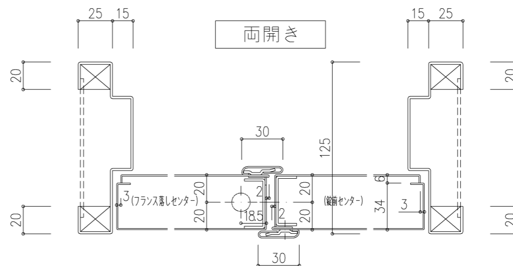
ST樑 目板付(R)
