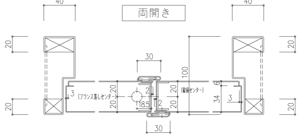
ST枠 目板付(R)
