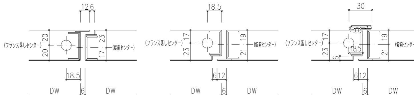
ST枠 目板一体 内開き(R) ST枠 目板一体 外開き(R) ST枠 目板付A(R)
