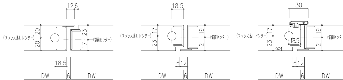
ST枠 目板一体 内開き(R)
