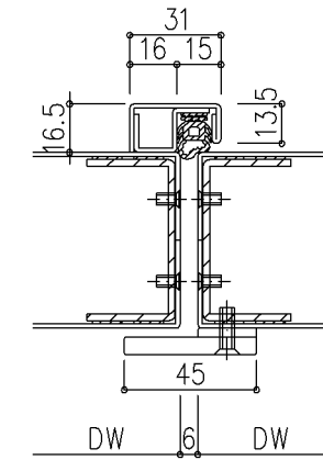
本図ハ右勝手ヲ示シ左勝手ハ左右対称トスル
