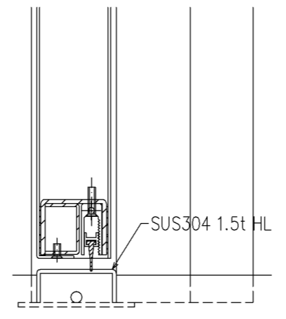
親子, 片側常閉両開き用子扉
