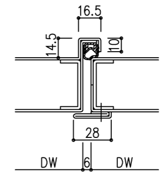
本図ハ右勝手フホシ左勝手ハ左右対称トスル
