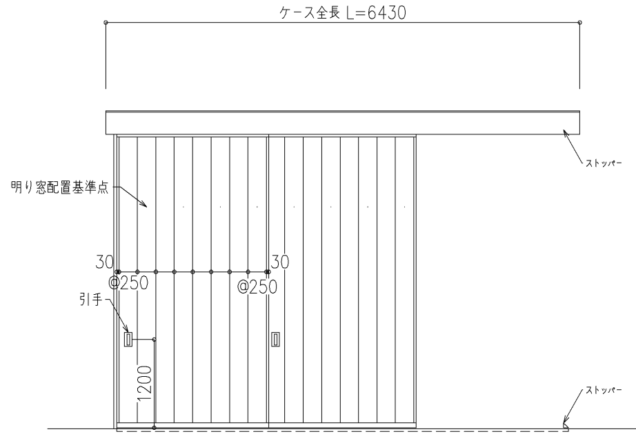
外観図
