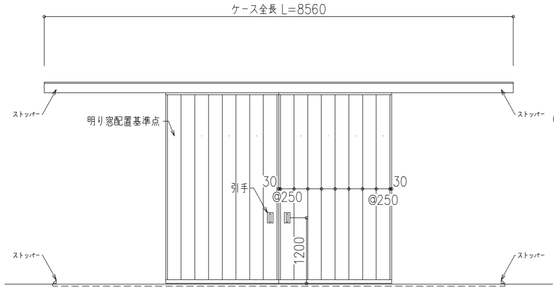
外観図
