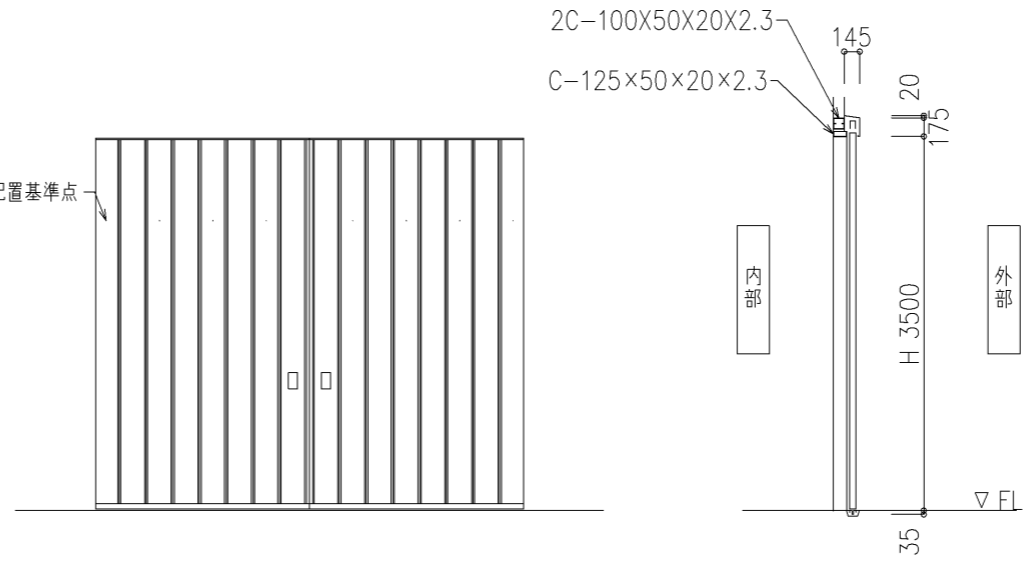
内観図
