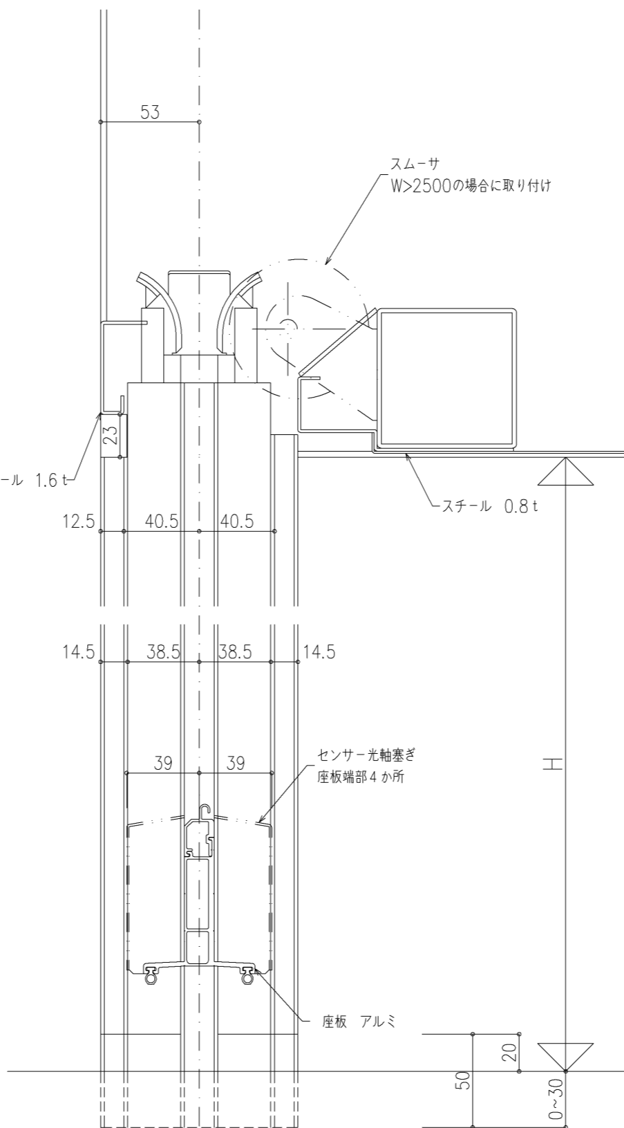
スチールケース詳細図
