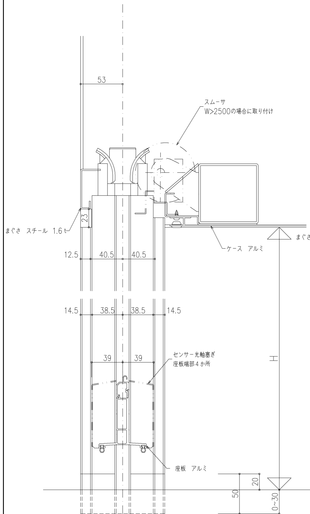
アルミケース詳細図
