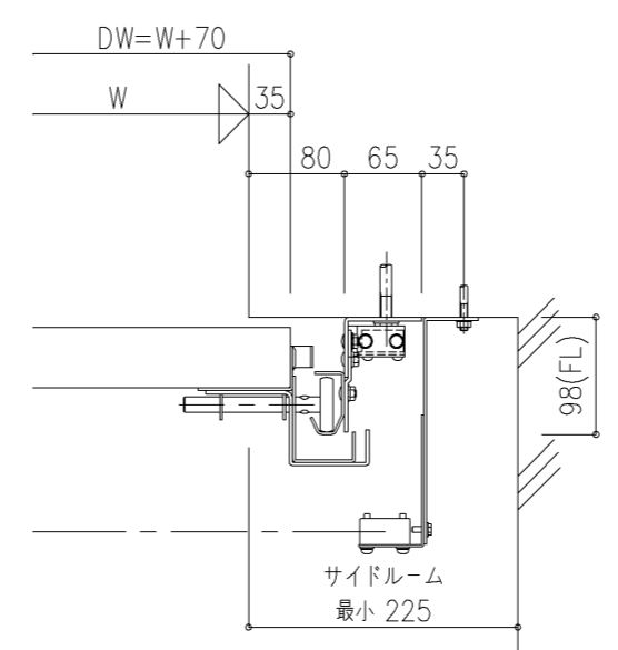
ガイドレール納まり詳細
