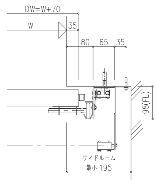
ガイドレール納まり詳細
