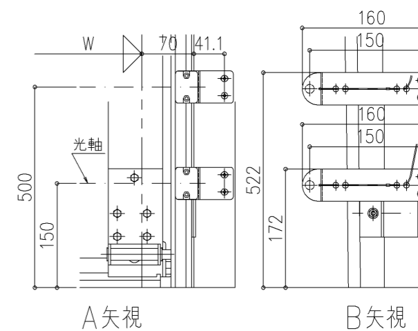
光電スイッチ部詳細
