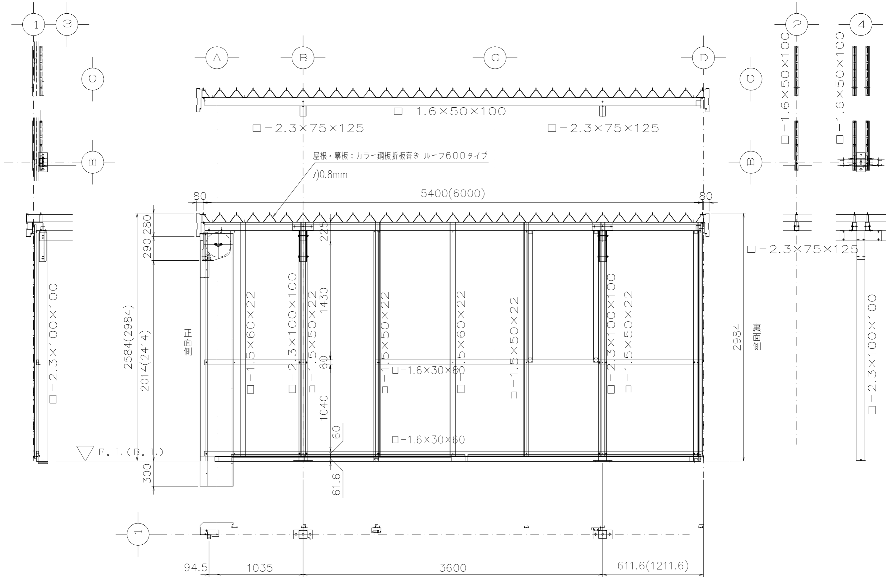
カポレージG-2S型(確認申請用) 1・2台用構造図
