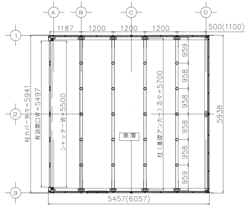
平面図 S = 1 / 50
