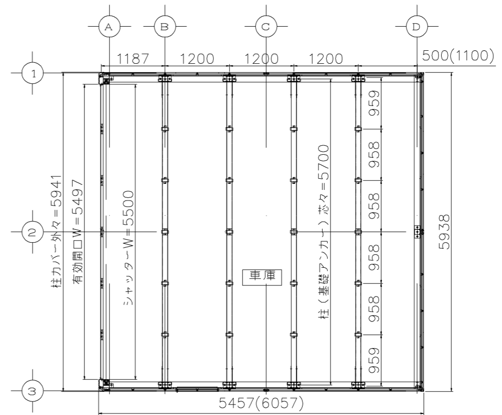
平面図 S = 1 / 50
