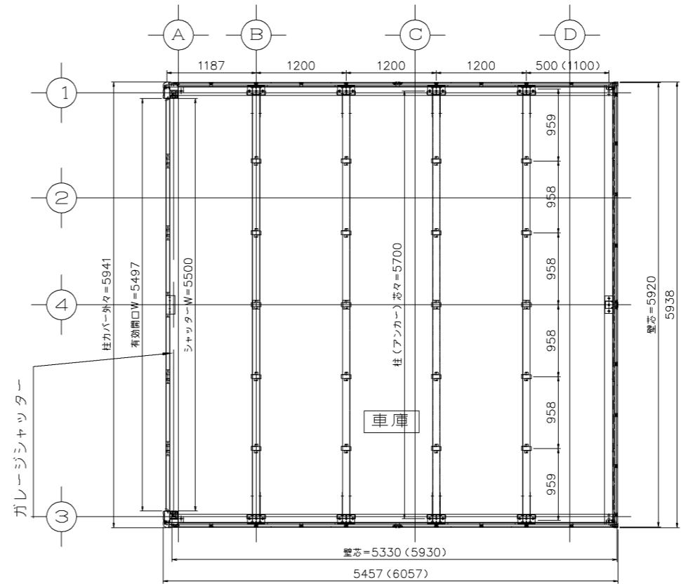
平面断面図 S = 1 / 50
