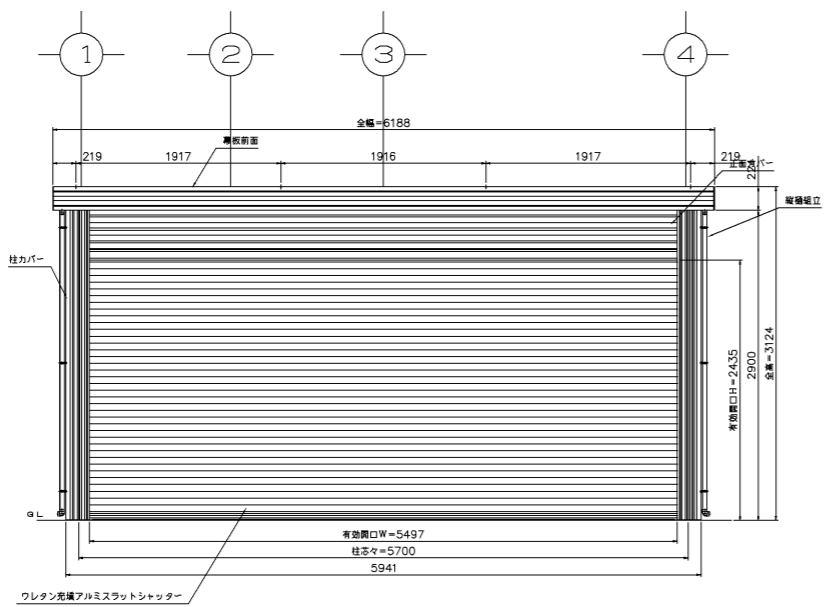
西立面図 S = 1 / 50
