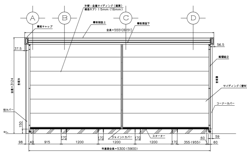
南(北)立面図 S = 1 / 50
