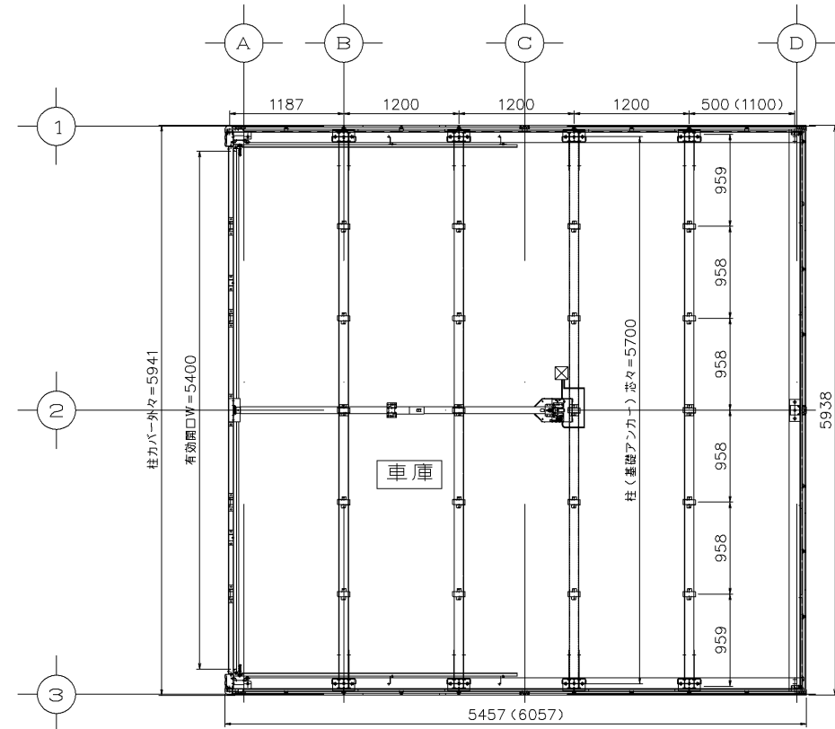
平面図 S = 1 / 50
