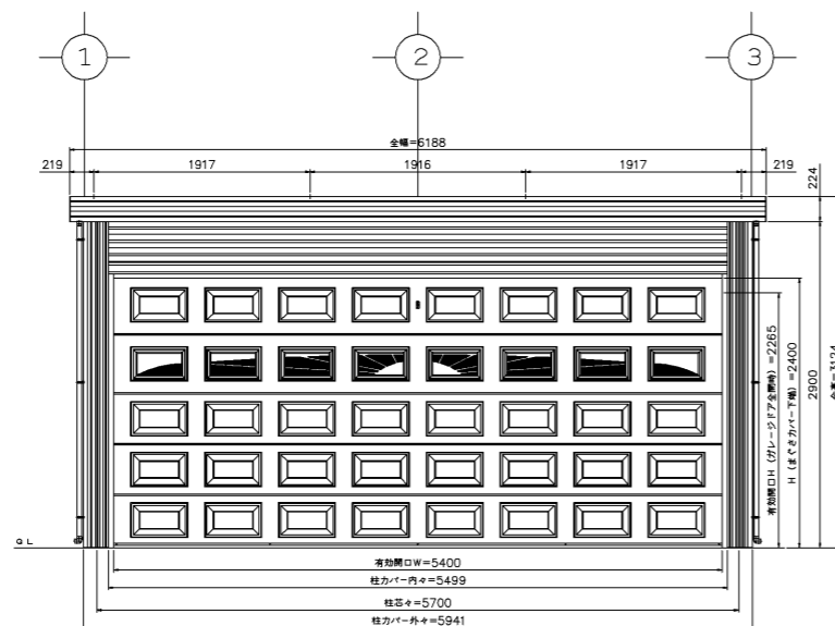
西立面図 S = 1 / 5 0
