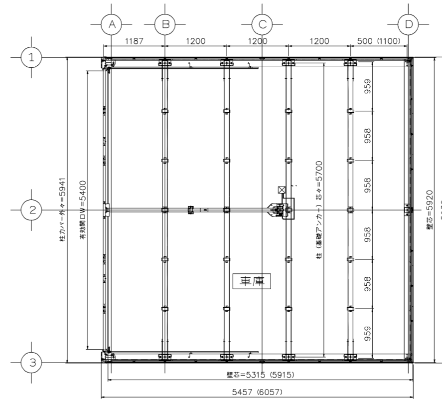
平面断面図 S = 1 / 5 0
