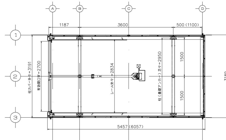
平面図 S = 1 / 50
