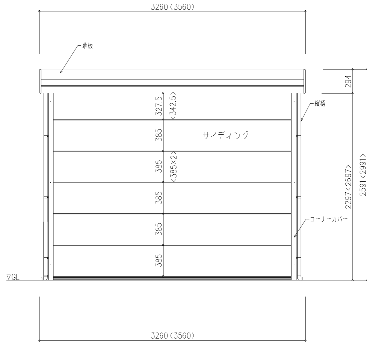
後面図
