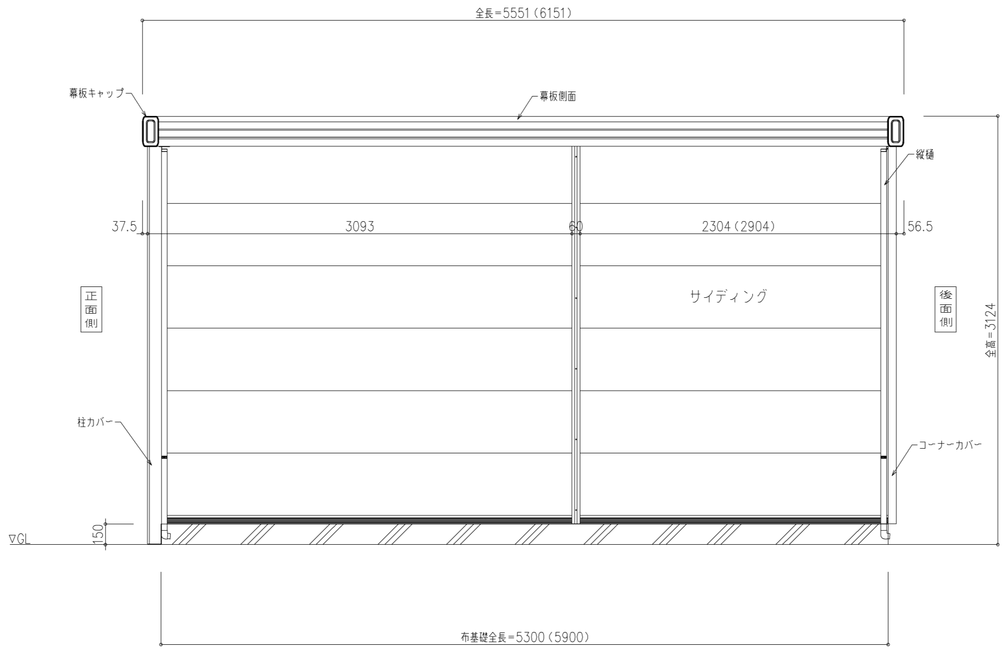
側面図
