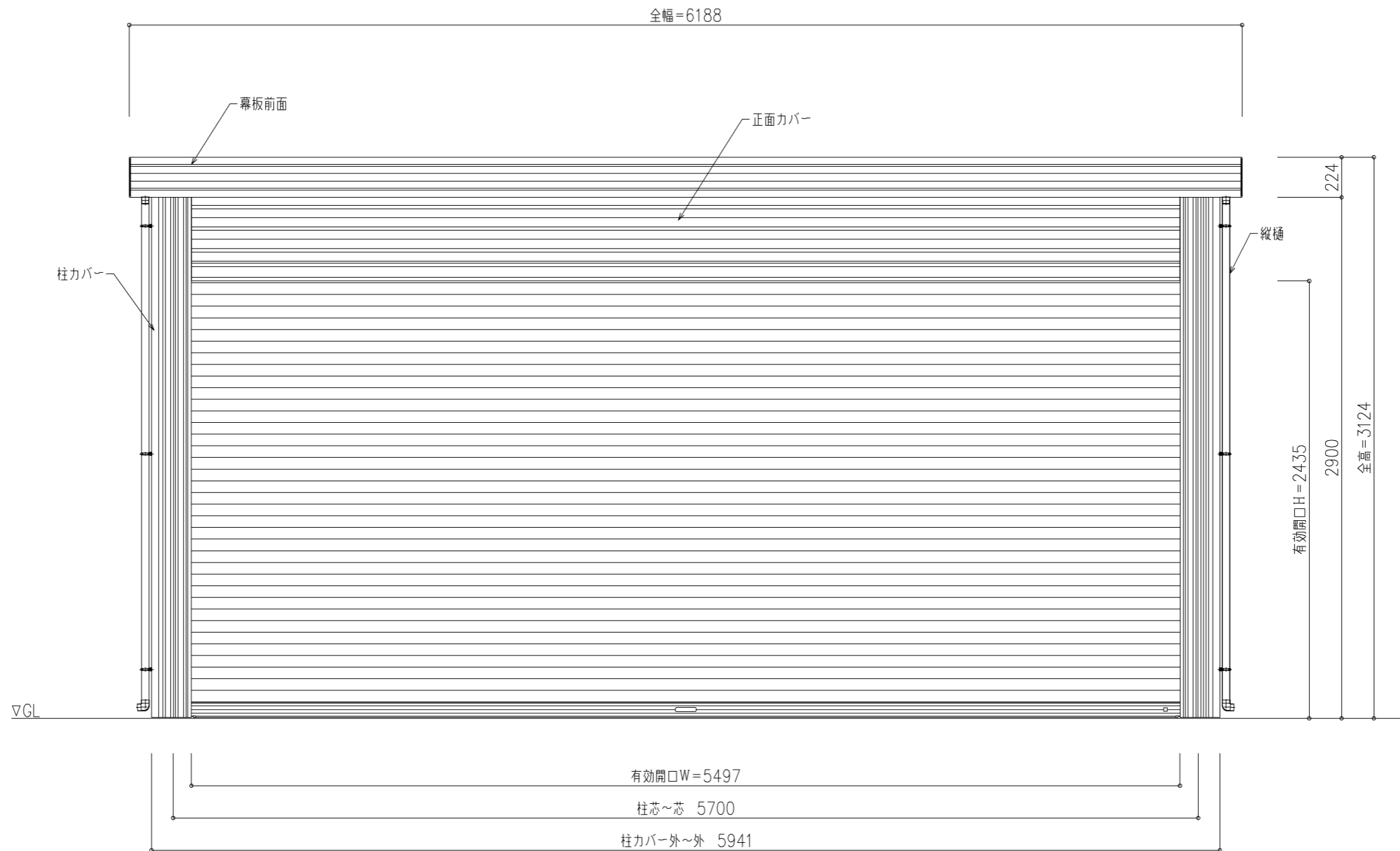
正面図
