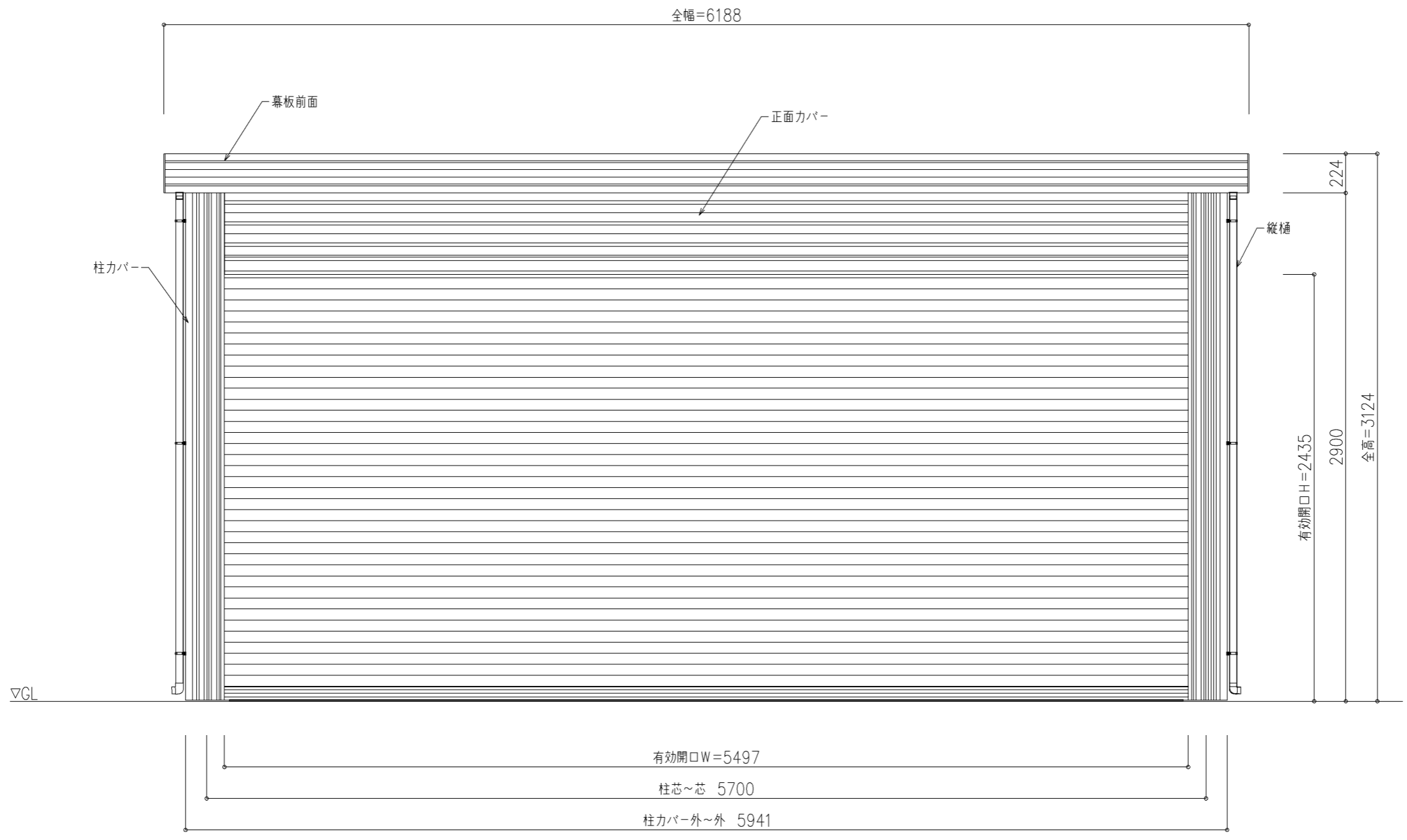
正面図
