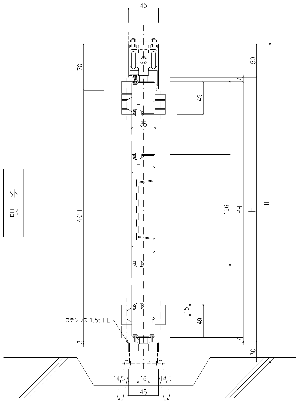
ダブルかまち1本
