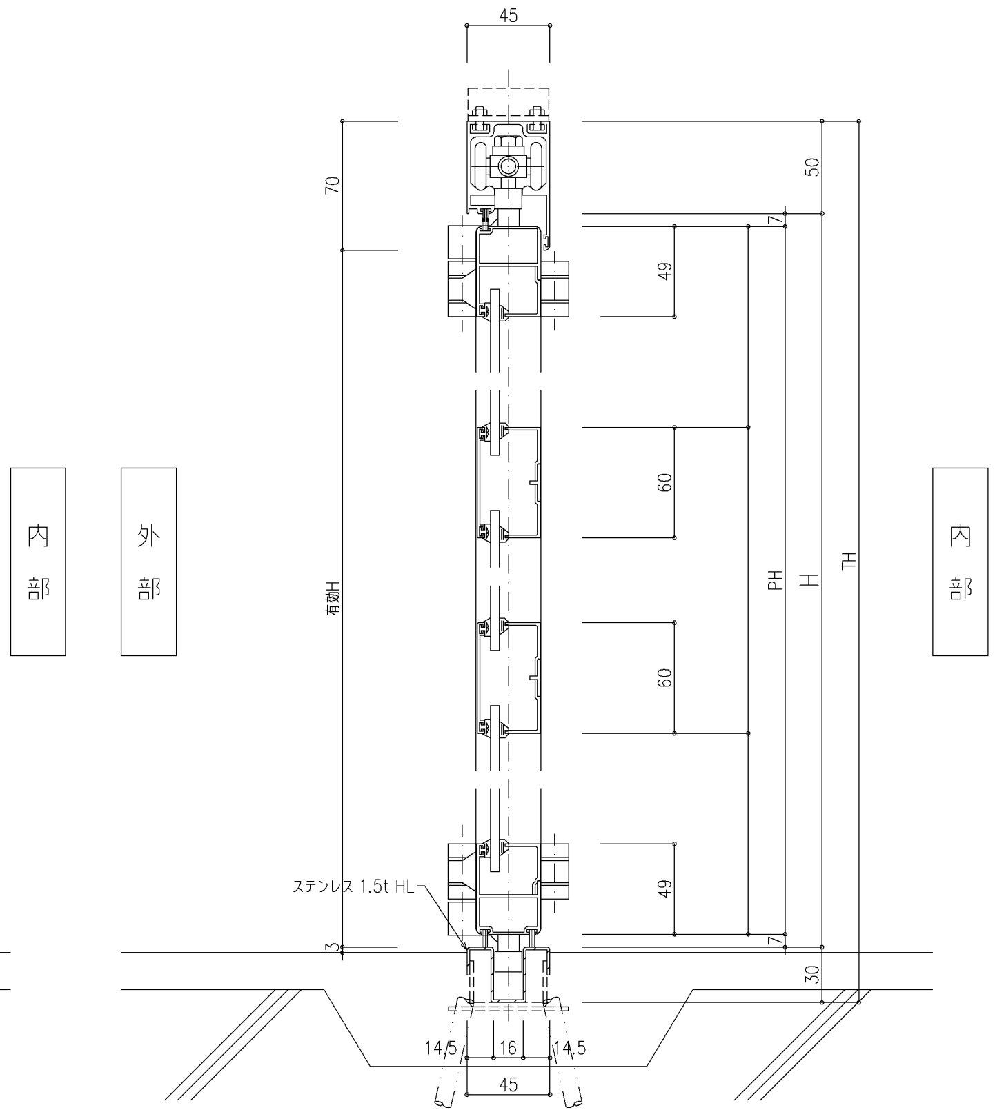
シングルかまち2本(1本)
