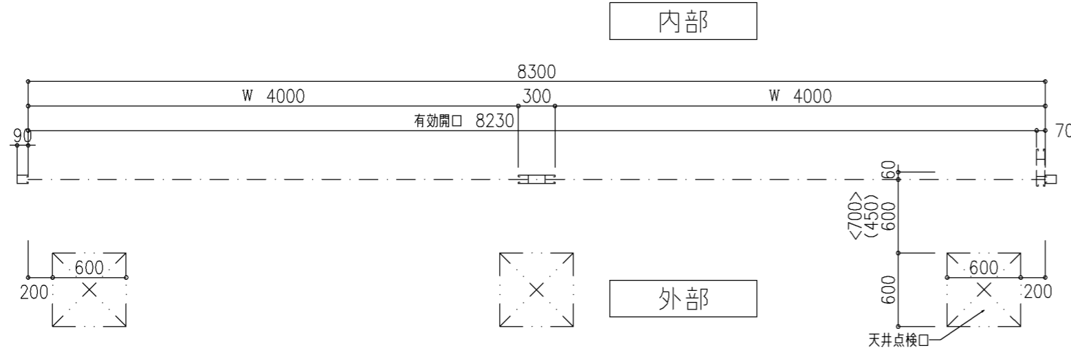
クリアード (Sタイプ) 可動中柱タイプ 外付け納まり
