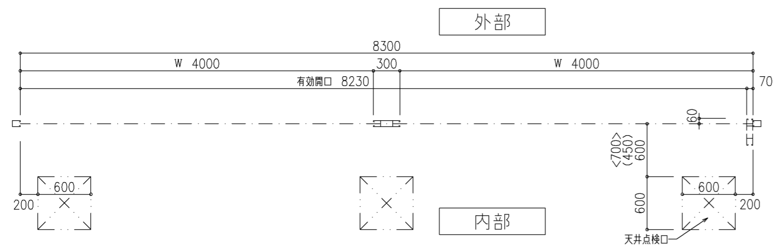
クリアード (Sタイプ) 可動中柱タイプ 内付け納まり
