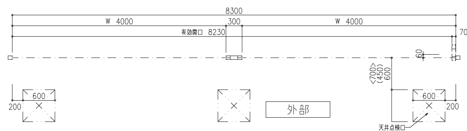
クリアード (Sタイプ) 可動中柱タイプ 外付け納まり
