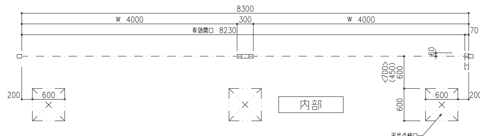
クリアード (Sタイプ) 可動中柱タイプ 内付け納まり
