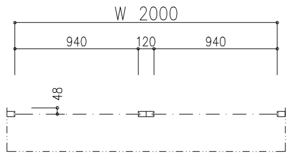
二連納まり
