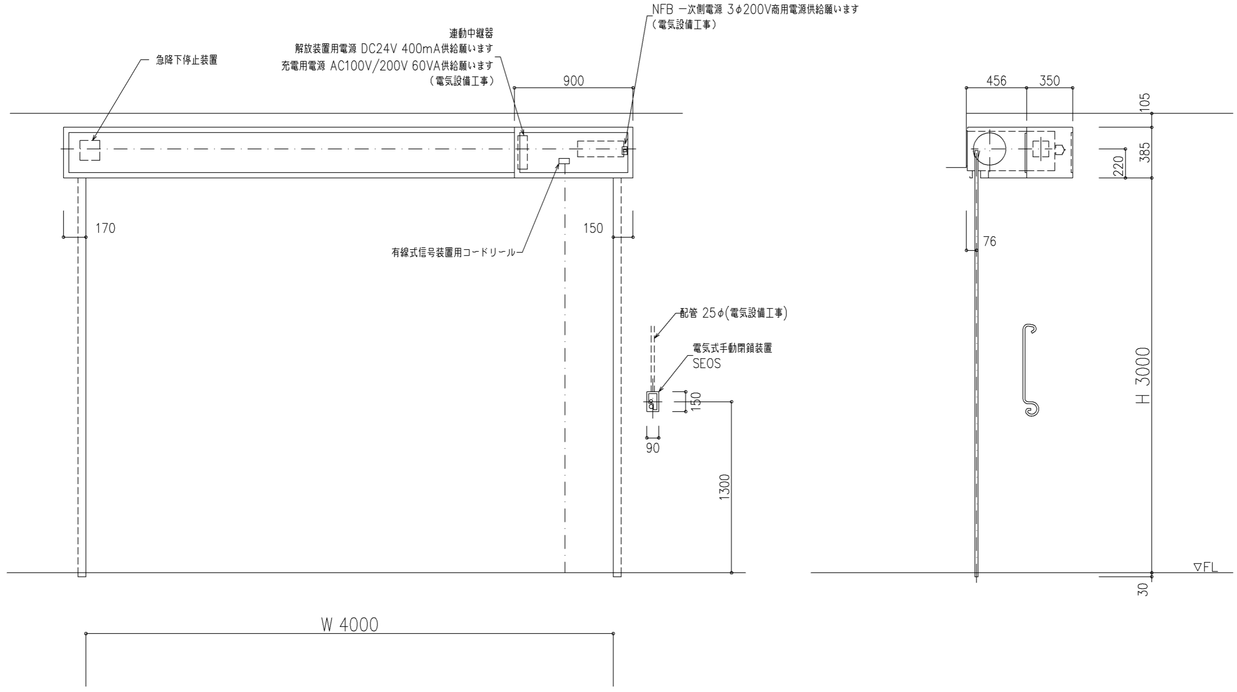
設計範囲 (F6スラット限定)
